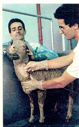
O emprego do fósforo radioativo sobre amostras de sangue, saliva e fezes revela como se processa o desenvolvimento de microorganismos no rúmen do animal.
